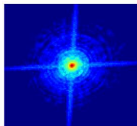
哈勃
