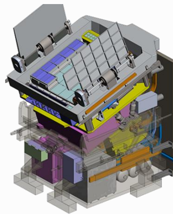
巡天模块
